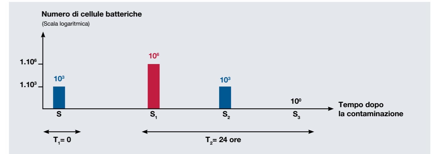
Carica batterica dopo la contaminazione del pavimento
